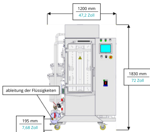
VORDERANSICHT
